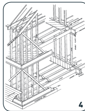
4. Sistema Platform Frame precursore del sistema a pannelli portanti.
