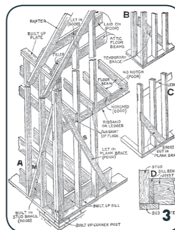
3. Sistema costruttivo a graticcio e montanti BalloonFrame.
